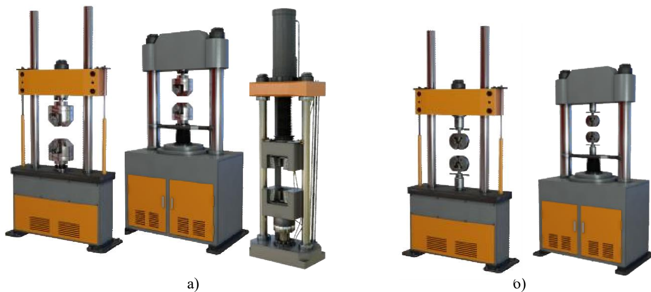
Рисунок 3 – Общий вид машин
